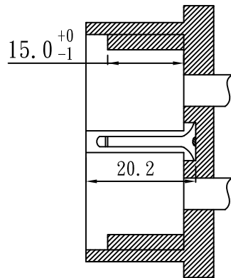
A--A(Broken)
